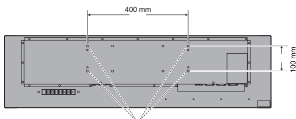
Interface de montage VESA (M6)
