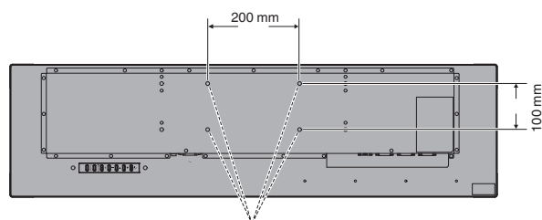
Interface de montage (M6)
