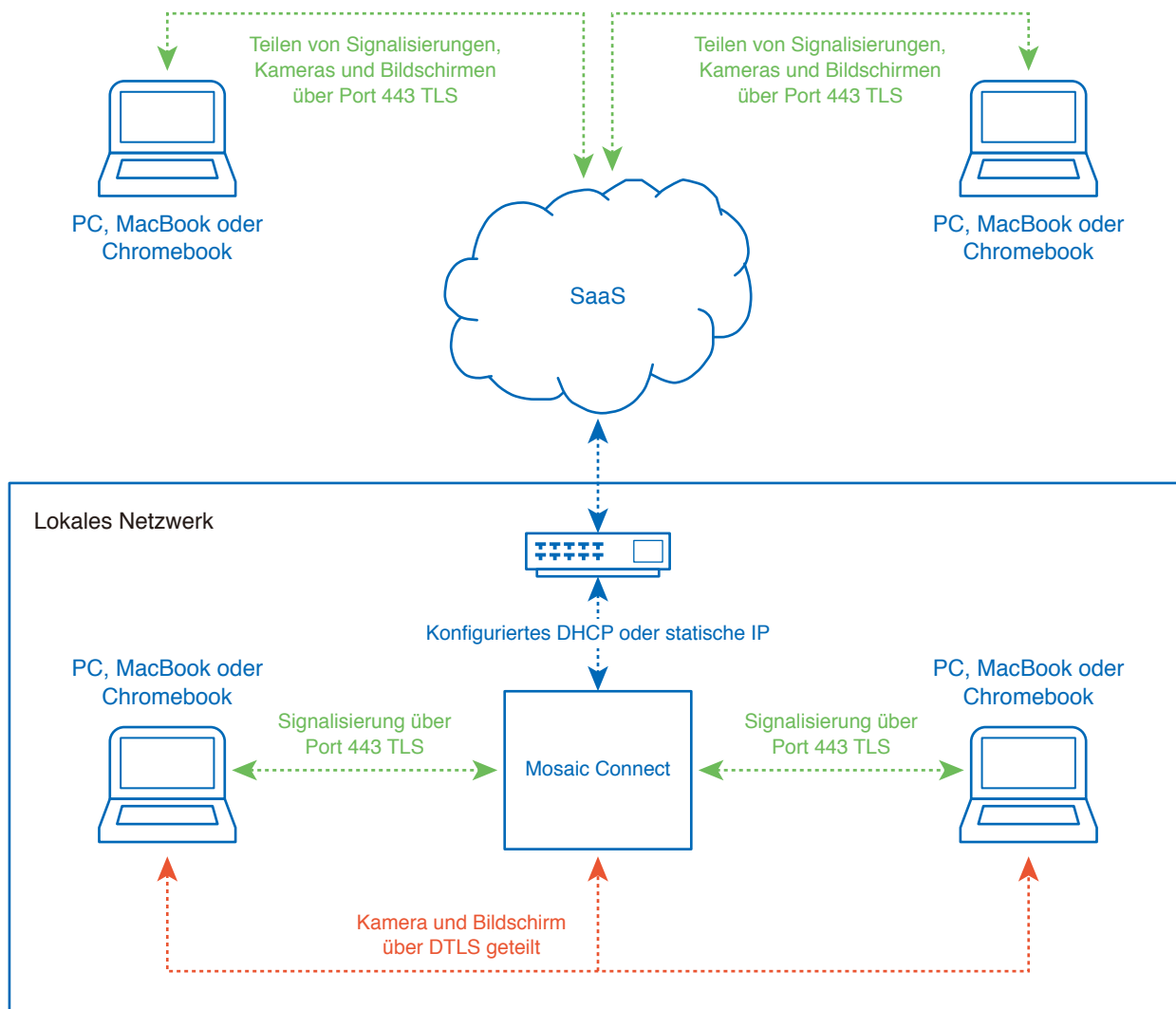
Abbildung 3. Netzwerkarchitektur von Mosaic Connect, interne und externe Verbindungen.
