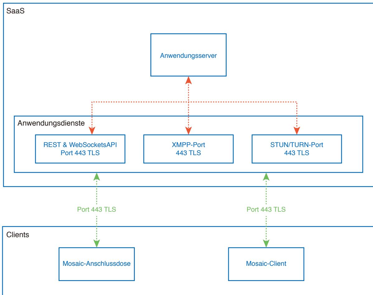
Abbildung 1. Mosaic Connect-Architektur
