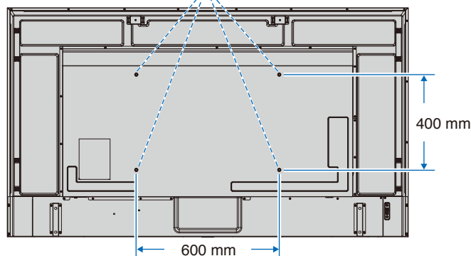
Монтажный интерфейс VESA (M8)
