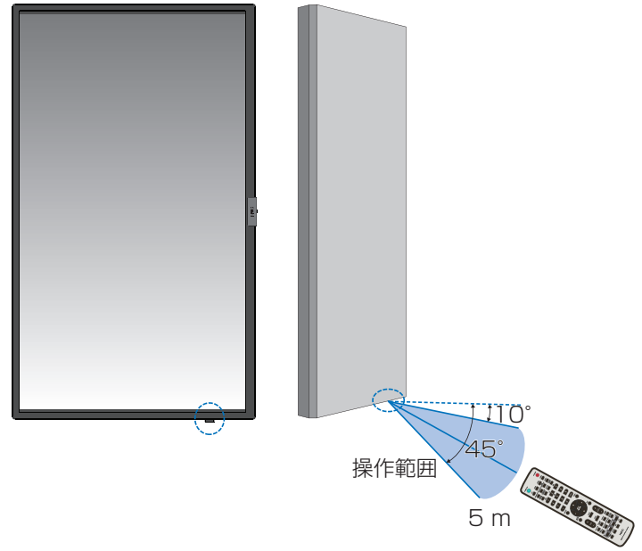
縦型設置時のリモコン操作範囲
