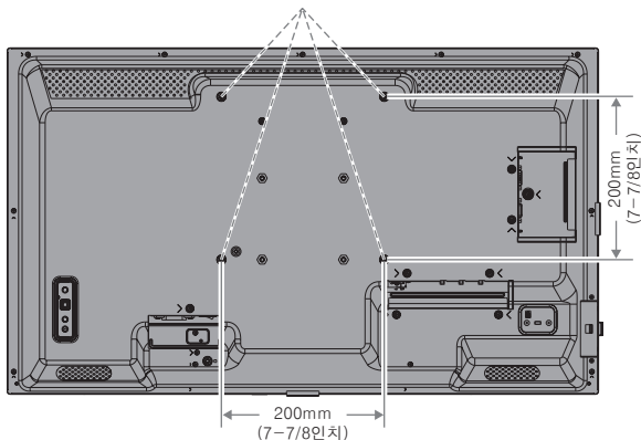
설치 접속면 (M4)
