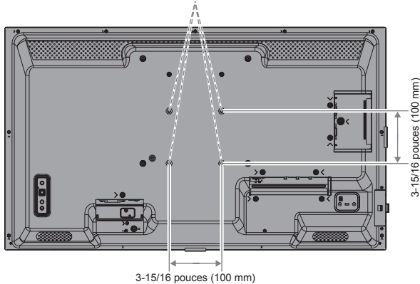
Interface de montage (M4)
