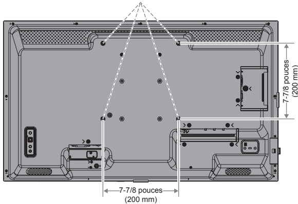
Interface de montage (M4)
