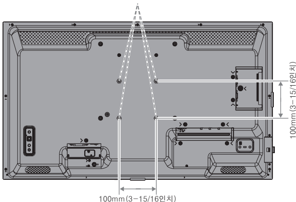
설치 접속면 (M4)
