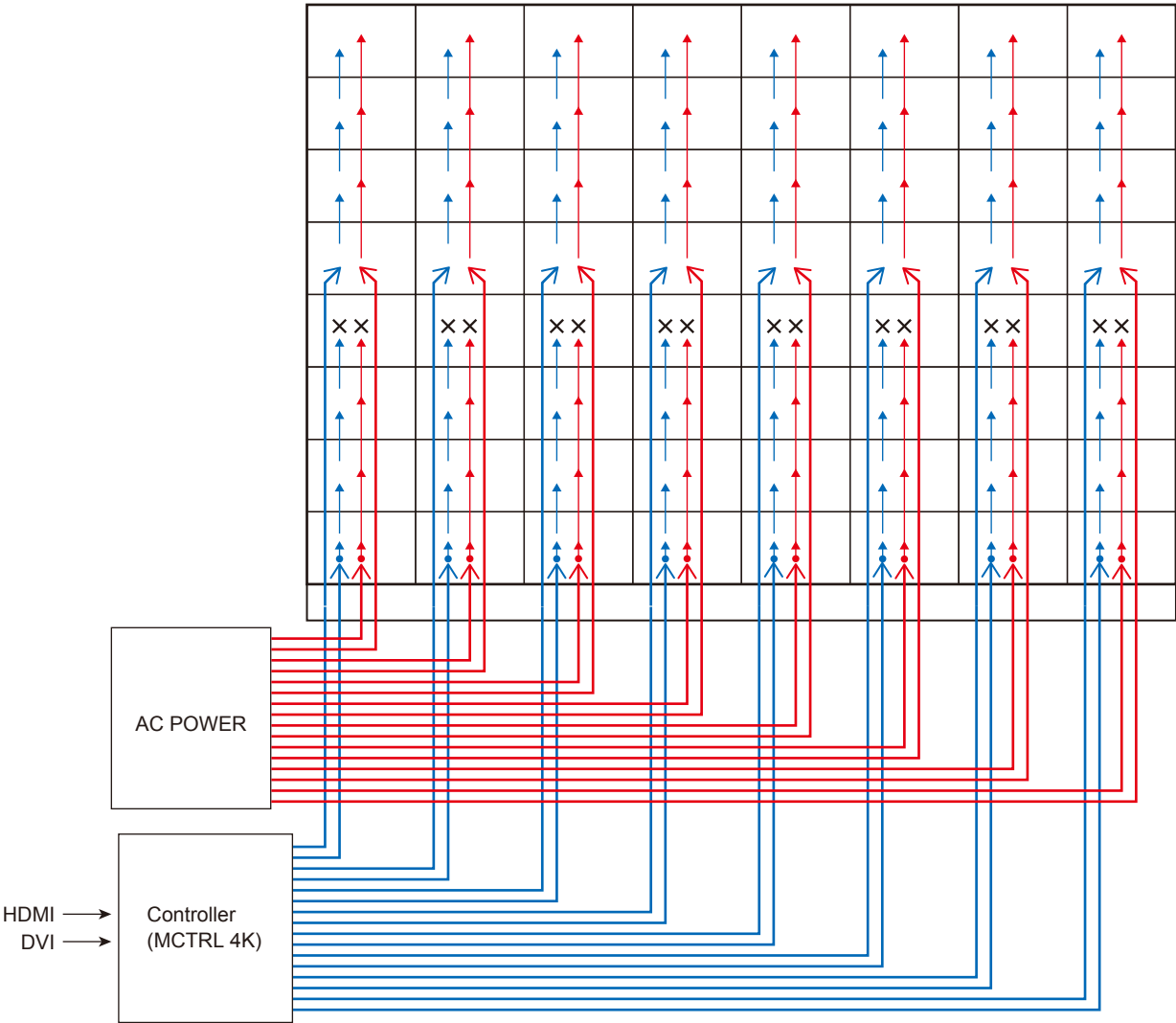
8 × 8 のフレームセット (1.2 mm ピッチ)
