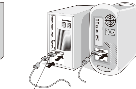
Adaptador para Macintosh
