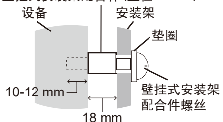
壁挂式安装架配合件 (直径 14 mm)
