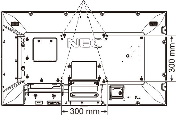
VESA 安装接口 (M6)
