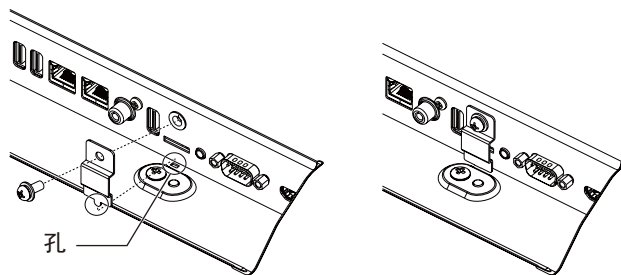
microSD 卡盖已装好。
