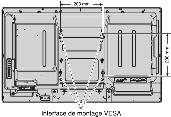
Interface de montage VESA
