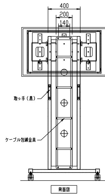
背面図
