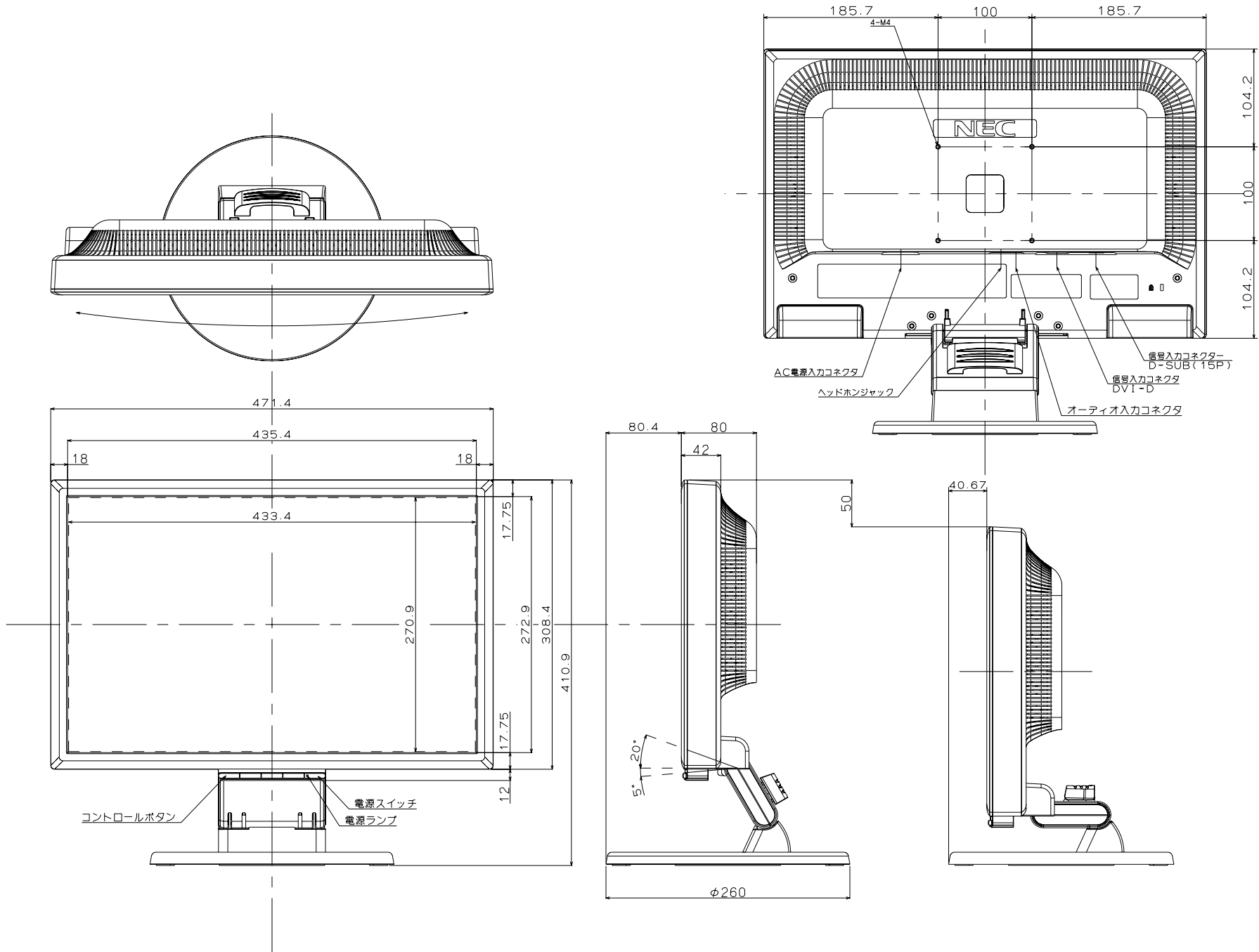
LCD205WXM 外観図
