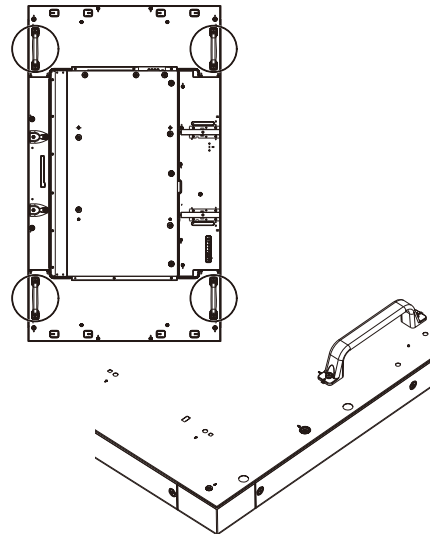
縦型設置時
