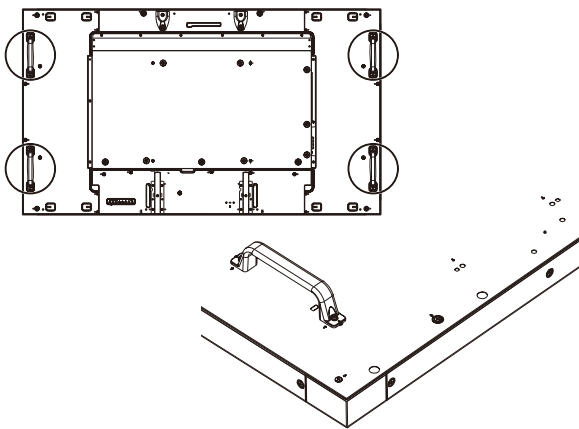
横型設置時
