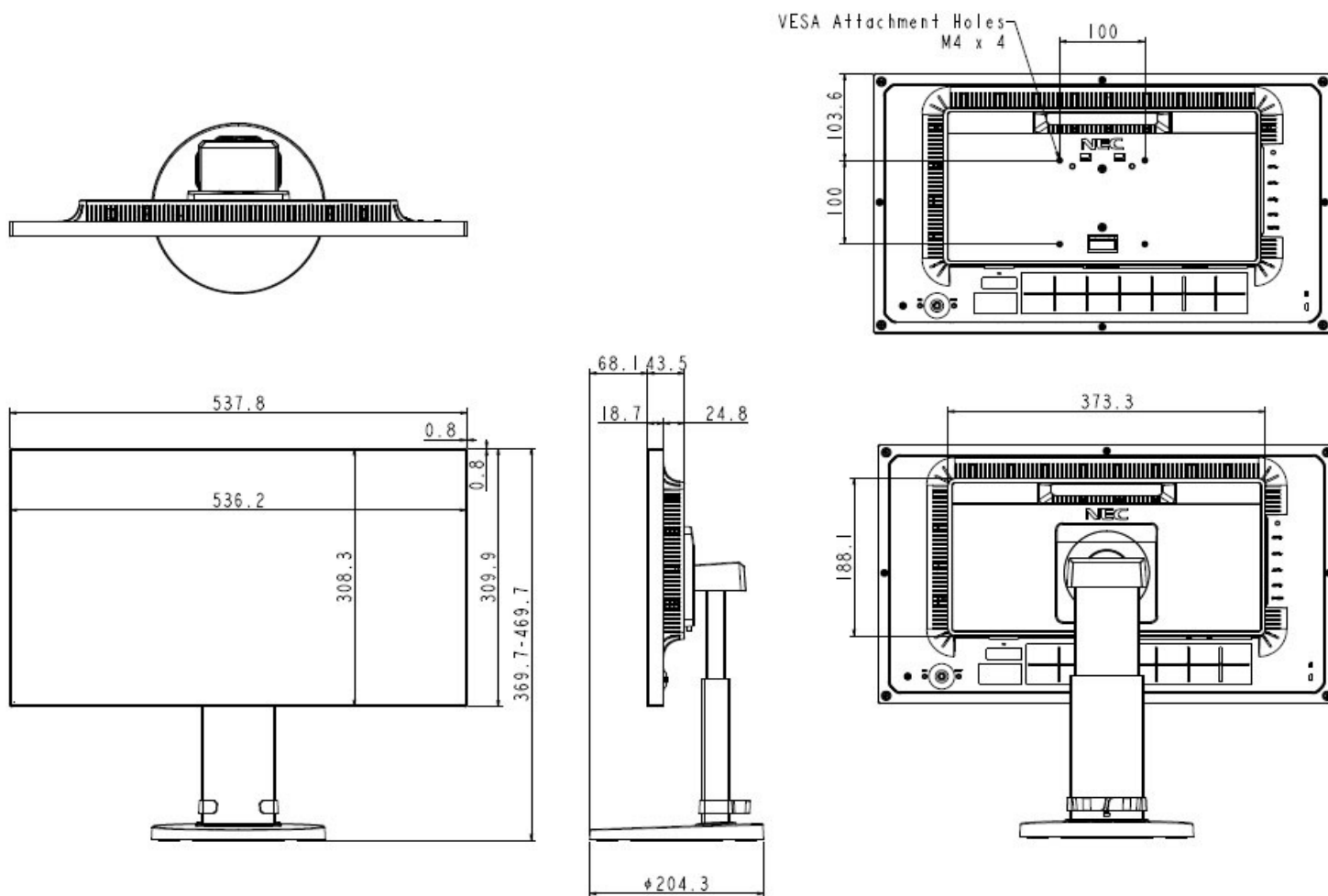
外形寸法図(mm)
