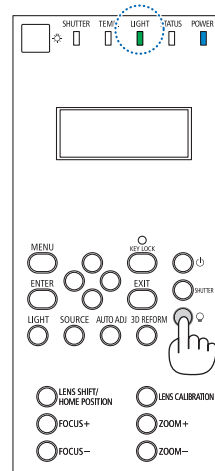
LIGHT 指示灯
