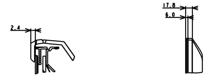
SECTION V0-V0 SCALE 1:1
