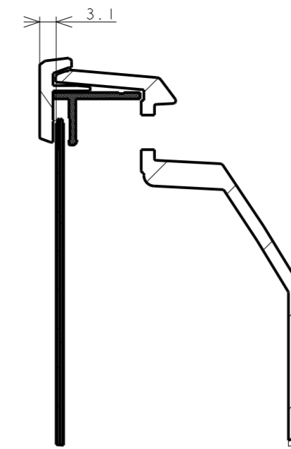
SECTION V0-V0 SCALE 1:1
