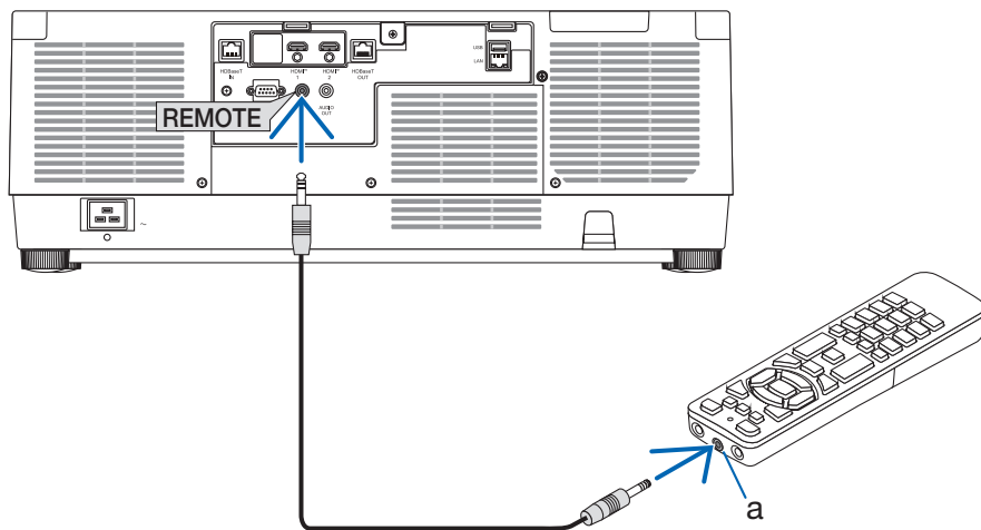
a: Fernbedienungsbuchse
