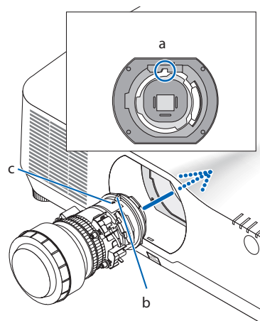
a: Προεξοχή / b: Εγκοπή / c: Βέλος
