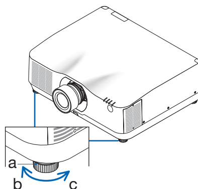
a: Πόδι με δυνατότητα κλίσης / b: Πάνω / c: Κάτω
