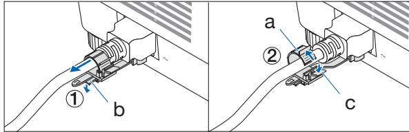
a: 클램퍼 / b: 손잡이(전원 코드 스토퍼) / c: 손잡이(클램퍼)
