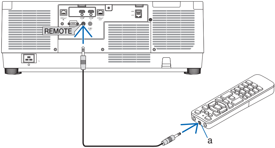
a：遠程控制插孔
