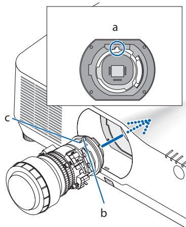
a: 導引槽/b: 突出部分/c: 箭頭
