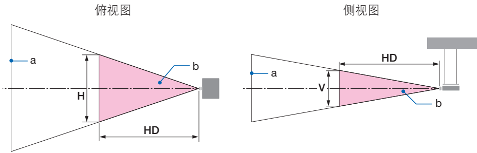
a: 屏幕 / b: 危害区域
