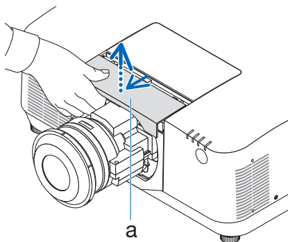
a: 镜头罩
