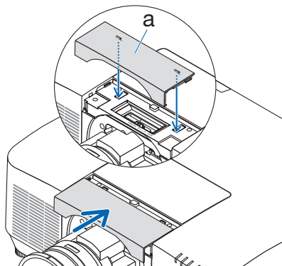
a: 镜头罩
