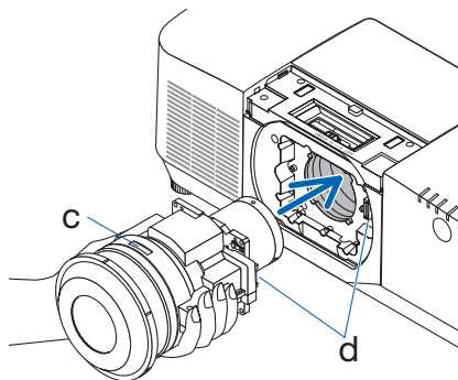
c: 板 / d: 接头
