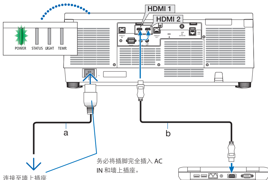
a：电源线（随附）/ b：HDMI线（未随附）
