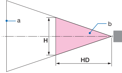
Üstten görünüm
