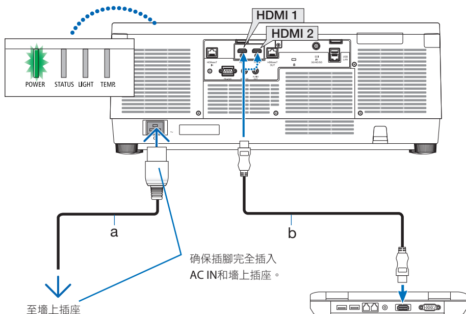
a：電線（隨附）/ b：HDMI線（未隨附）
