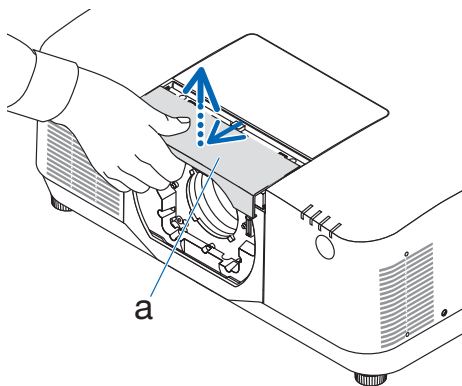
a: 镜头罩
