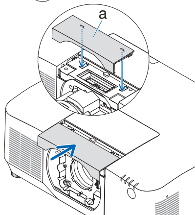
a: 镜头罩
