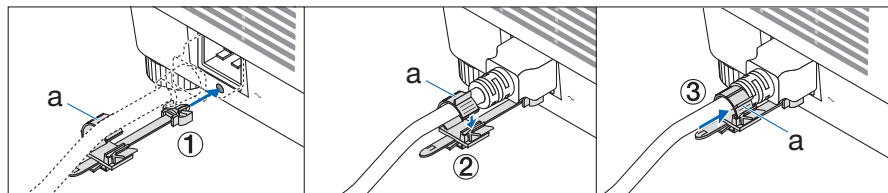
a: 夹具
