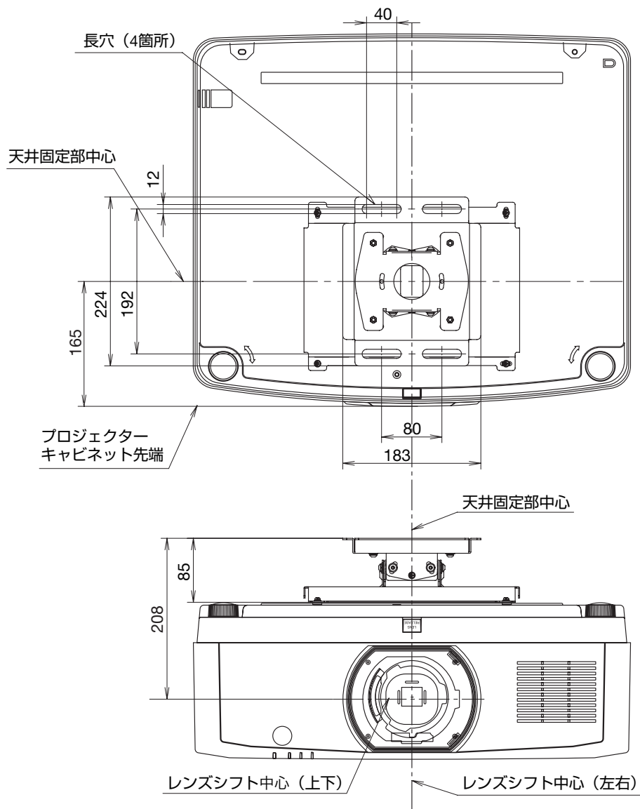
天井設置面寸法図（単位：mm）
