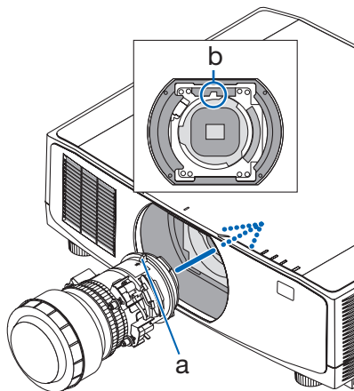
a: 凸起 / b: 导向槽口
