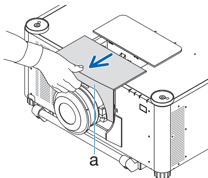
a: 镜头罩
