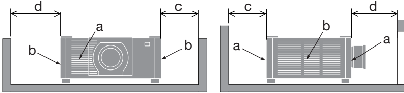
a: ilmanottoaukko/b: ilmanpoistoaukko/c: vähintään 20 cm/ d: vähintään 30 cm
