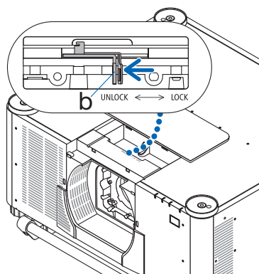
b: Leva di blocco obiettivo
