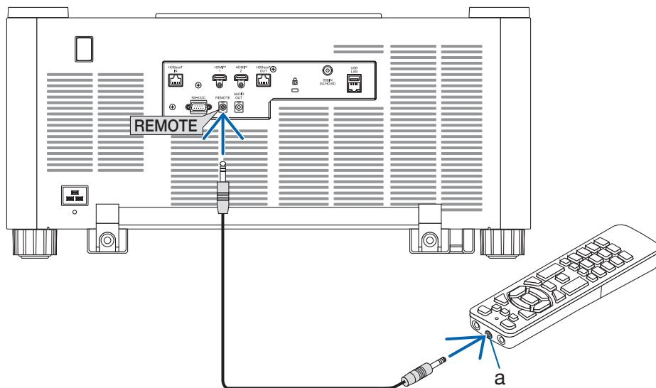
a: Jack remoto
