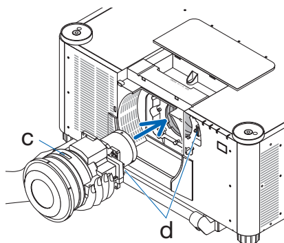
c: Piastra/d: Connettore
