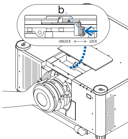
b: Leva di blocco obiettivo
