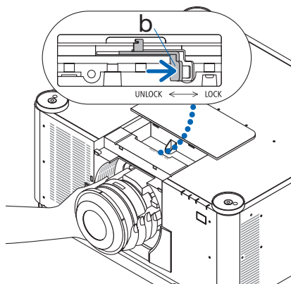
b: Leva di blocco obiettivo
