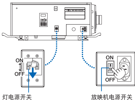
灯电源开关
