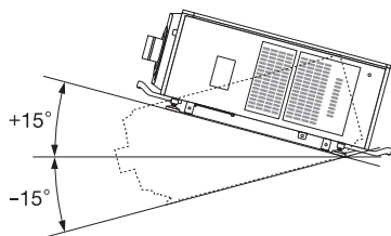
床置きで設置する場合
