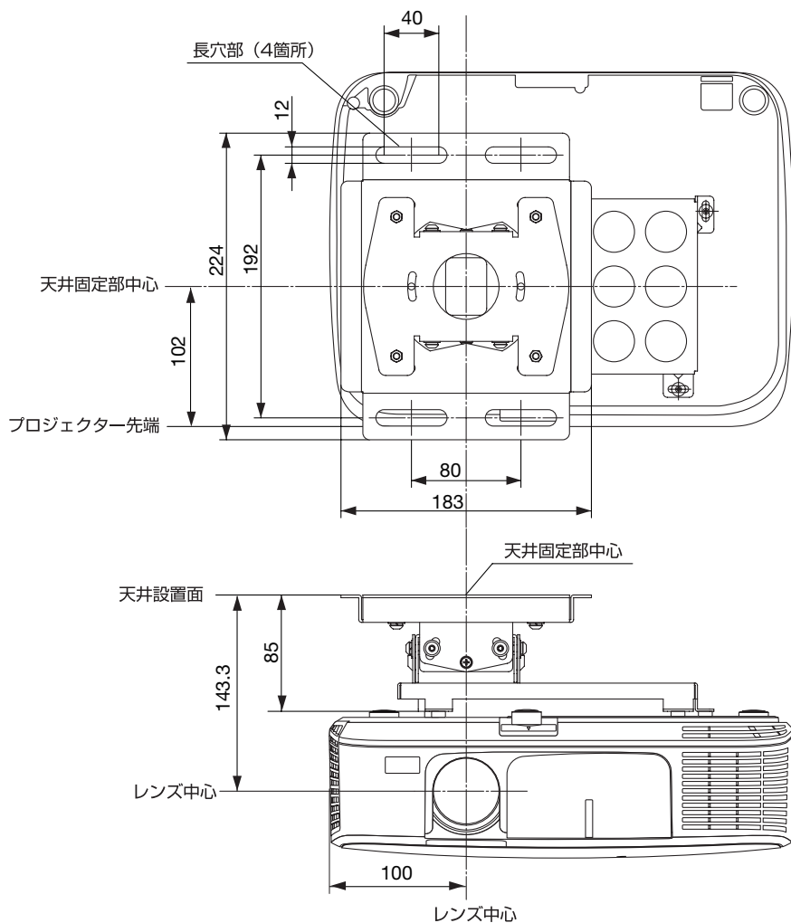
天井設置面寸法図（単位：mm）
