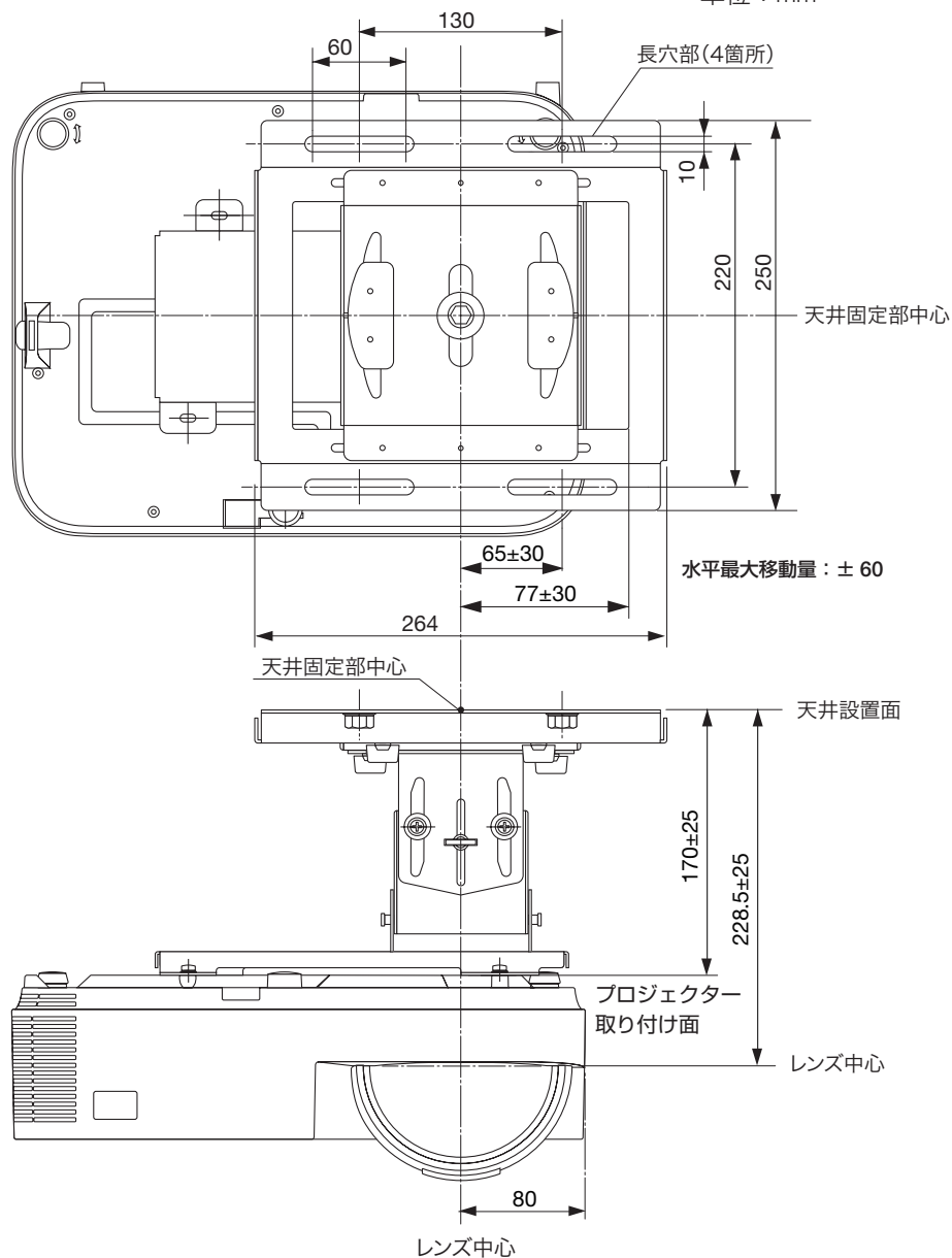
天井設置面寸法図
