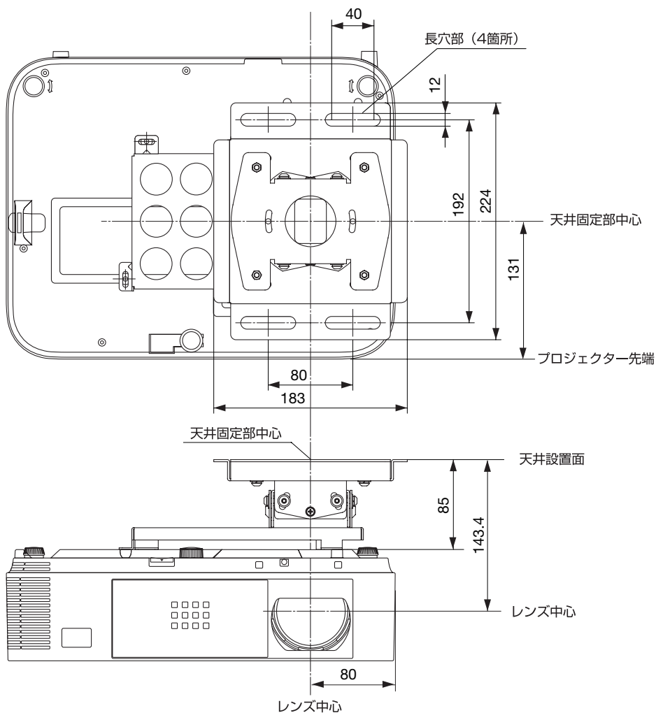
天井設置面寸法図（単位：mm）
