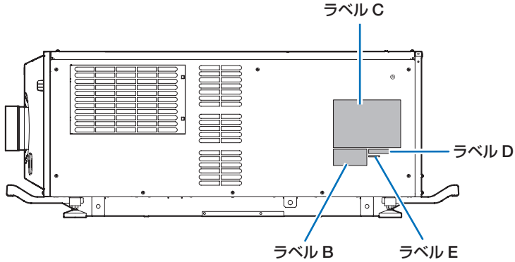
ラベル B Laser Explanatory Label (レーザー説明ラベル)
