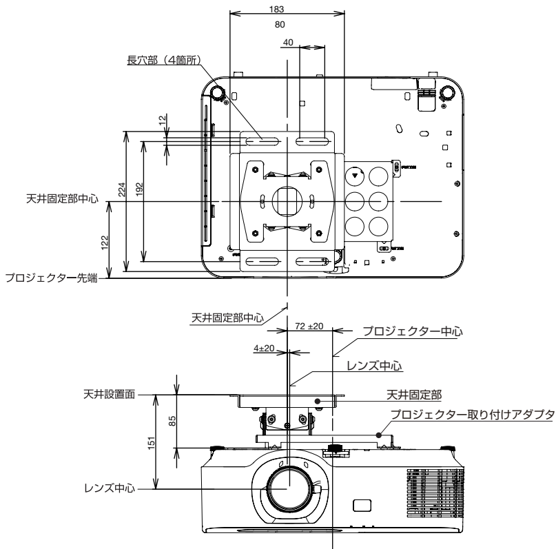
天井設置面寸法図（単位：mm）
